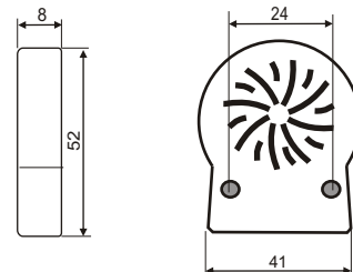
Рис.1. Габаритные и установочные размеры
