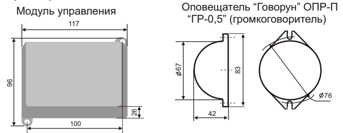
Рис.1. Габаритные и установочные размеры
