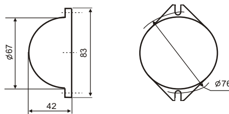
Рис.1. Габаритные и установочные размеры оповещателя
